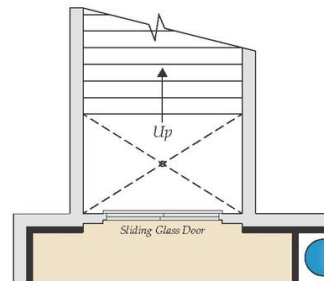
OPT. DOUBLE DOOR AREAWAY
